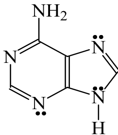
adenina
