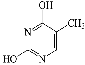
2,4-diossi-5-metil-pirimidina
