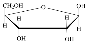
\beta -D-ribosio
