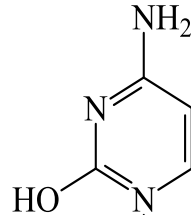
2-ossi-4-ammino-pirimidina
