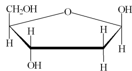
\beta -D-2-desossiribosio
